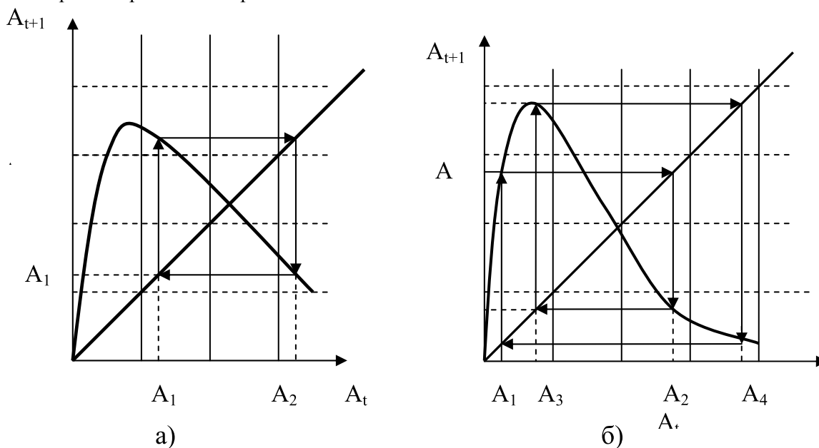
Рисунок 2- Динамическая спираль – циклы периода 2(а) и 4(б).
