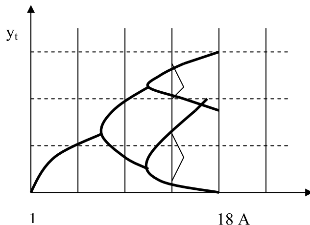
Рис.3 Бифуркционная диаграмма одномерного отображения
