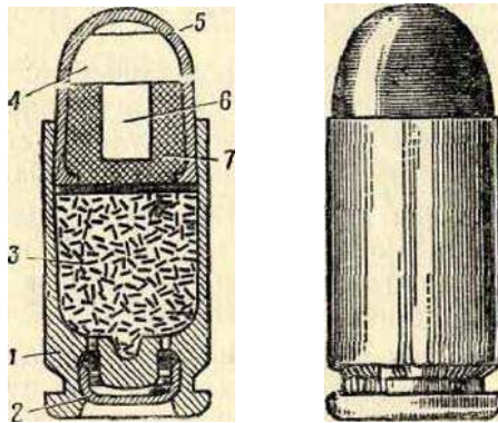
Рис. 20. Общий вид 9-мм пистолетного патрона и его устройство 1 :
