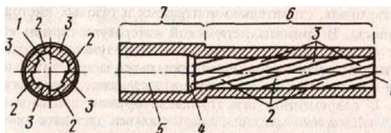
Рис. 13: Ствол нарезного оружия в продольном и поперечном разрезе 1 :
