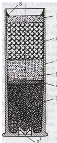
Рис. 21. Охотничий патрон в поперечном разрезе
