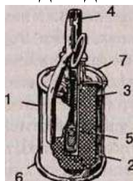
Рис. 23. Устройство ручной осколочной гранаты РГ-42 1 :
