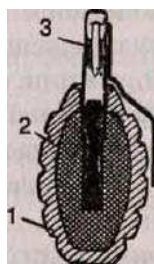
Рис. 24. Устройство ручной осколочной гранаты Ф-1:
