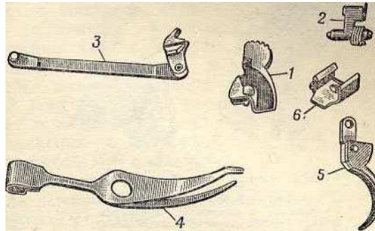
Рис. 18. Части ударно-спускового механизма 1 :
