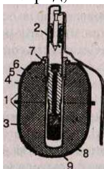
Рис. 25. Устройство ручной осколочной гранаты РГД-5
