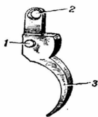
Рис. 27. Спусковой крючок 1 — цапфа; 2 — отверстие; 3 — хвост.
