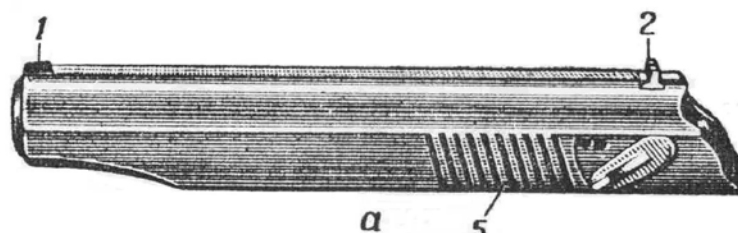
Рис. 17. Затвор (вид с левой стороны):
