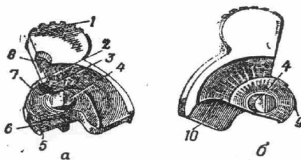
Рис. 24. Курок:
