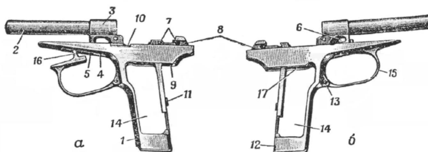
Рис. 41. Рамка со стволом и спусковой скобой:
