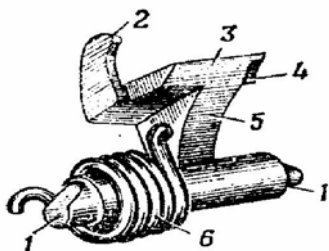
Рис. 25. Шептало:
