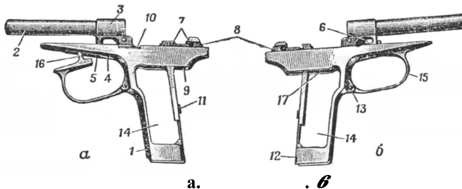
Рис. 16. Рамка со стволом и спусковой скобой: а – левая сторона; б – правая сторона: 1 – основание рукоятки; 2 – ствол; 3 – стойка для крепления ствола; 4 – окно для размещения спускового крючка и гребня спусковой скобы; 5 – гнезда для цапф спускового крючка; 6 – кривой паз для размещения передней цапфы спусковой тяги; 7 – гнезда для цапф курка и шептала; 8 - пазы для направления и движения затвора; 9 – окно для перьев боевой пружины; 10 – вырез для затворной задержки; 11 – прилив с отверстием для крепления рукоятки; 12 – вырез для защелки магазина; 13 – прилив с гнездом для крепления спусковой скобы; 14 – боковые окна; 15 – спусковая скоба; 16 – гребень для ограничения движения затвора назад; 17 – окно для выхода верхней части магазина.
