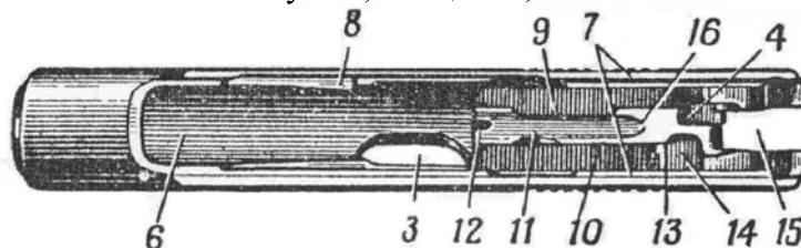
Рис. 18. Затвор (вид снизу):
