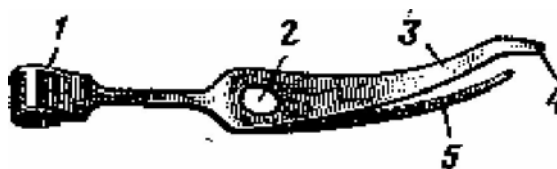
Рис. 28. Боевая пружина: 1 — защелка; 2 — отверстие; 3 — широкое перо; 4 — отбойный конец; 5 — узкое перо
