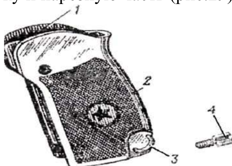
Рис. 29. Рукоятка с винтом: 1 — пазы; 2 — отверстие; 3 — антабка; 4 — винт
