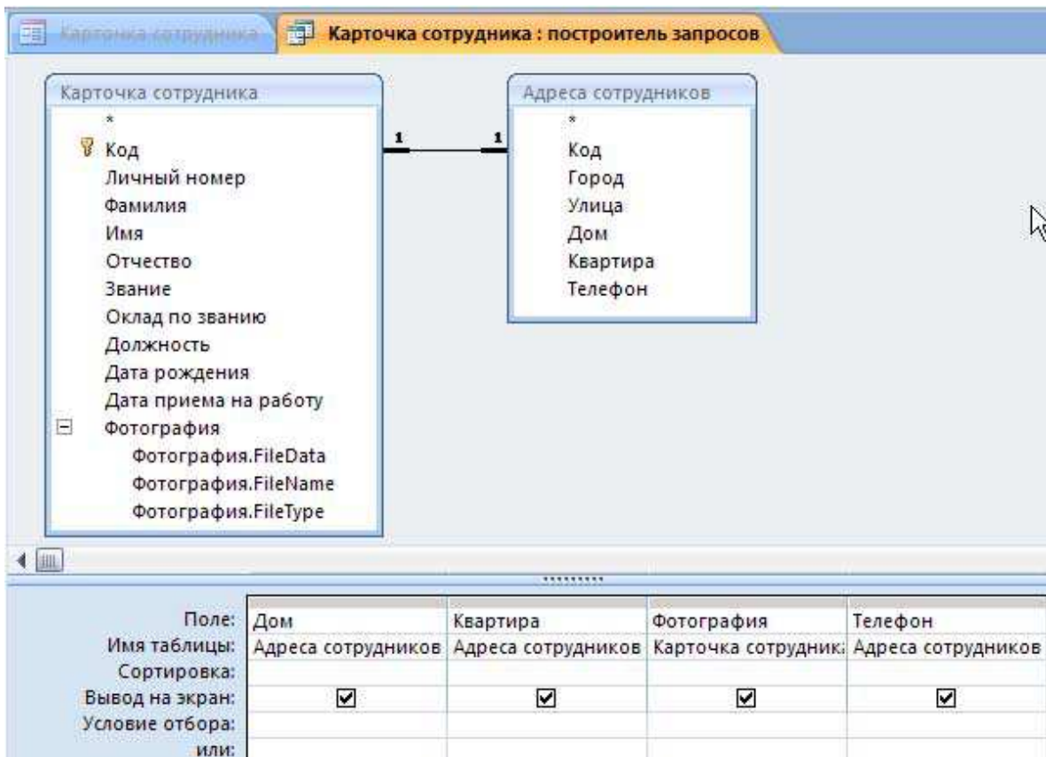
Рис.7.2. Окно построителя запросов
