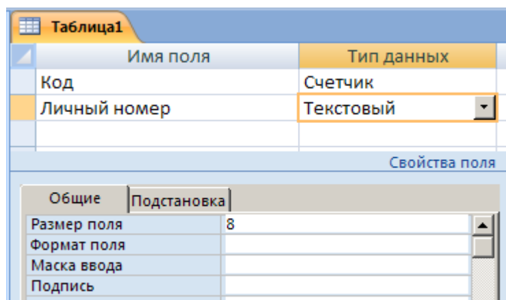
Рис. 2.4. Окно свойств поля Личный номер
