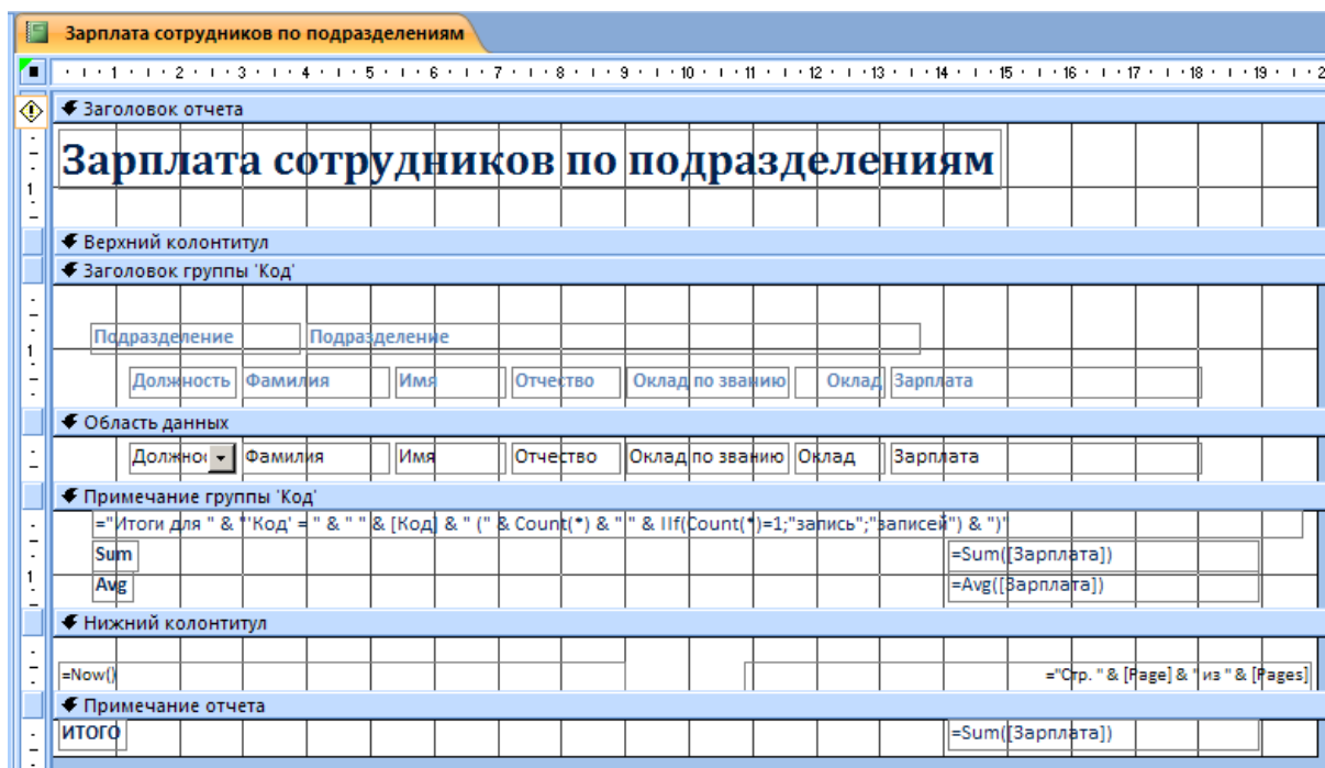
Рис.5.7. Конструктор отчета Зарплата сотрудников по подразделениям
