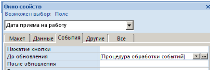
Рис.6.3. Свойства поля Дата приема на работу
