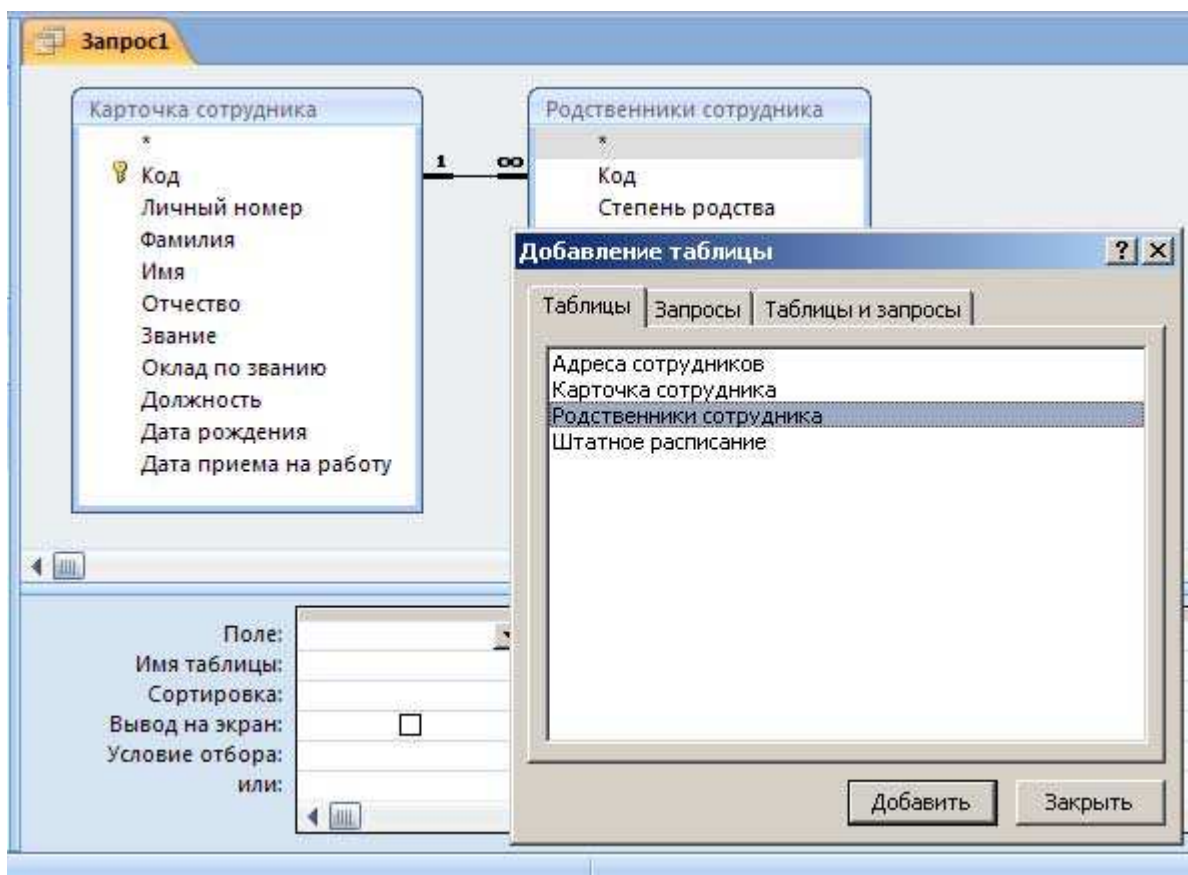
Рис.4.3. Добавление таблиц в конструкторе запросов
