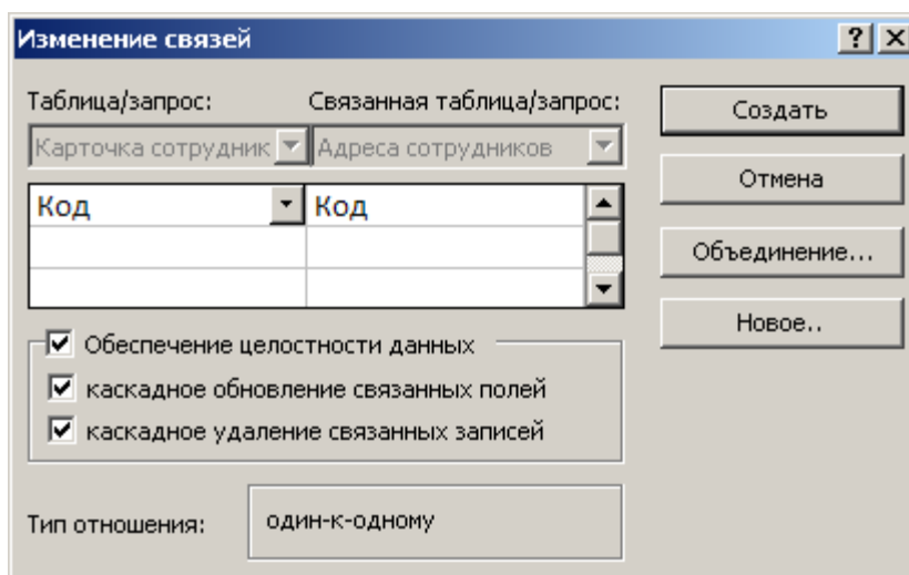
Рис.2.8. Параметры связи
