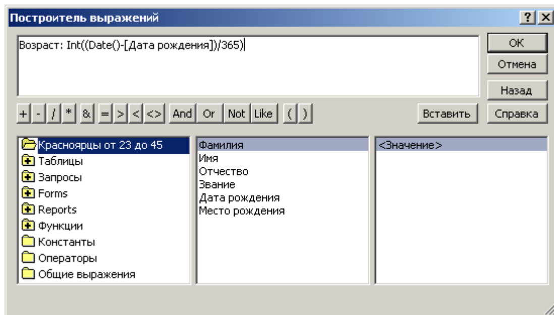
Рис.4.6. Построитель выражений
