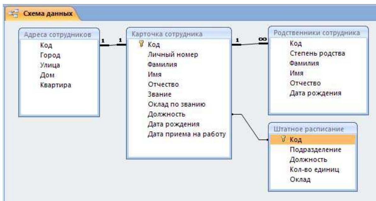
Рис.2.7. Схема данных
