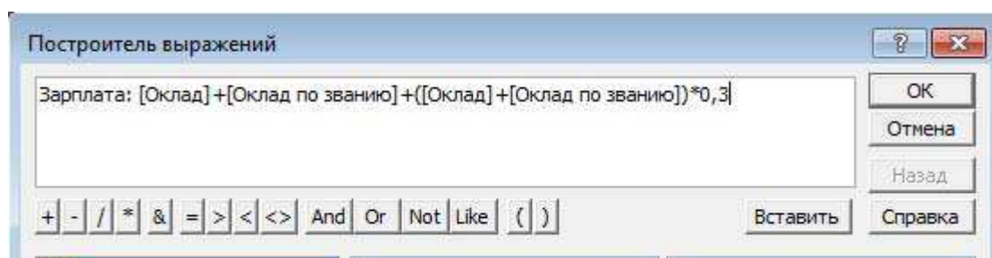
Рис.4.8. Выражение для вычислимого поля Зарплата
