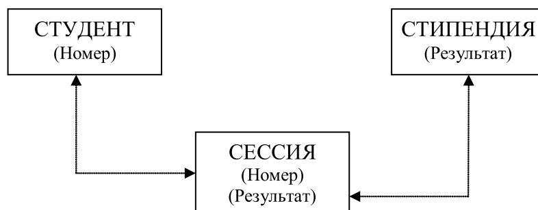
Рис.1.5. Пример реляционной модели
