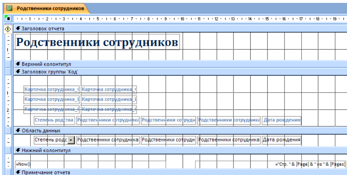
Рис.5.2. Конструктор отчетов
