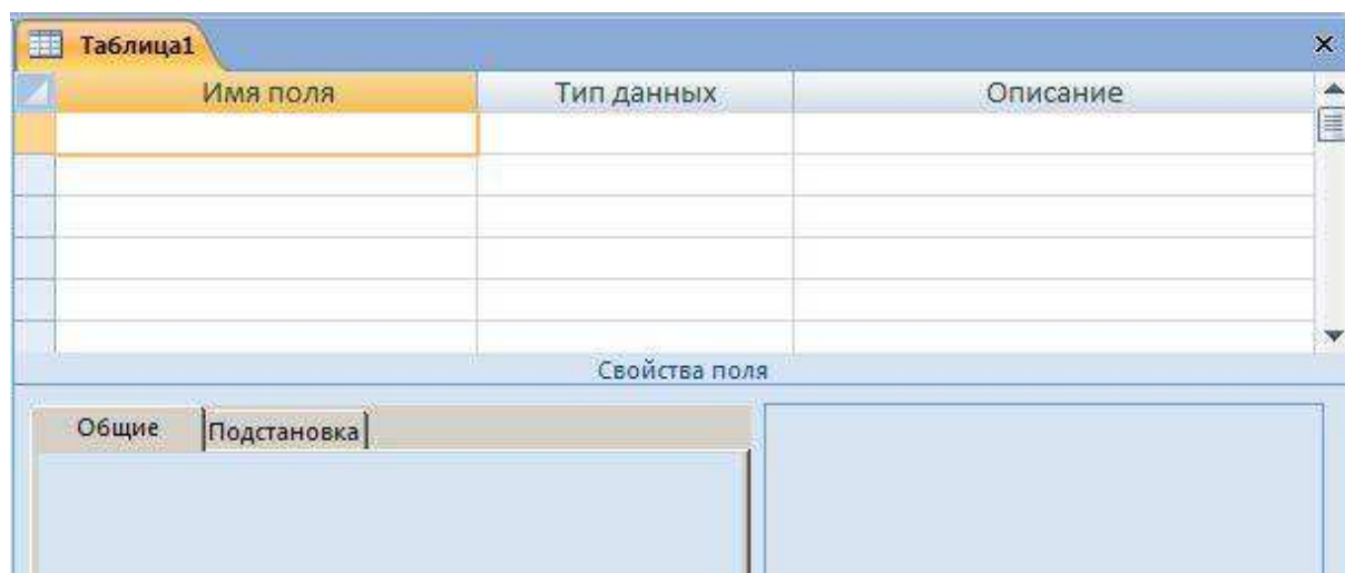
Рис.2.3. Конструктор таблиц
