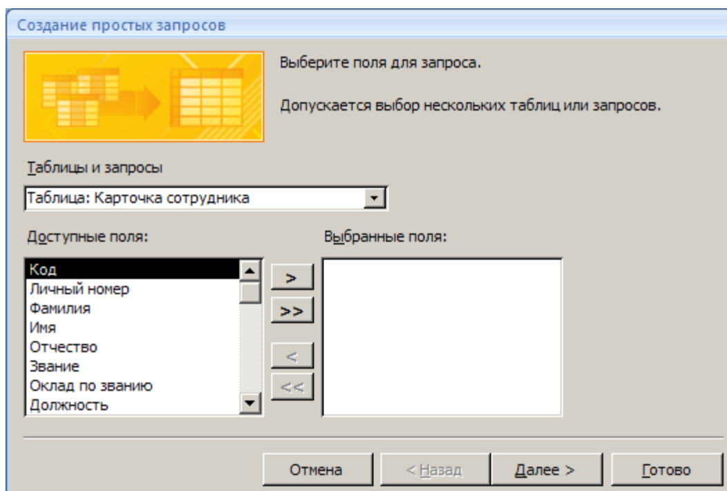
Рис.4.1. Мастер запросов
