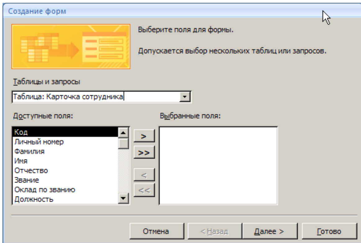
Рис.3.1. Мастер форм
