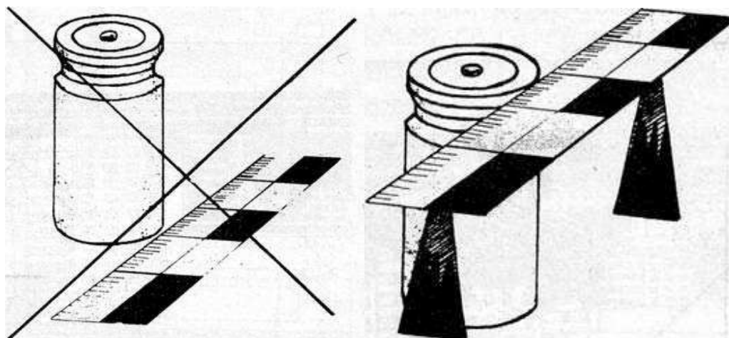
Рис. 9. Неправильное (слева) и правильное (справа) расположение криминалистической линейки при производстве детальной съемки объемных объектов
