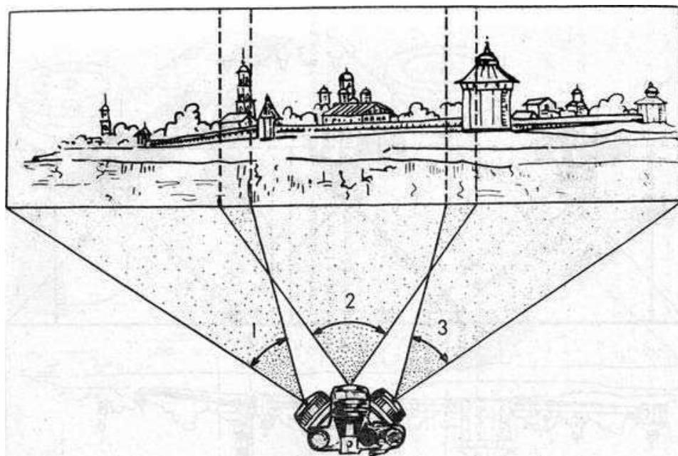
Рис. 8. Схема производства ориентирующей съемки методом круговой панорамы
