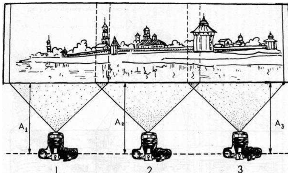
Рис. 7. Схема производства ориентирующей съемки методом линейной панорамы
