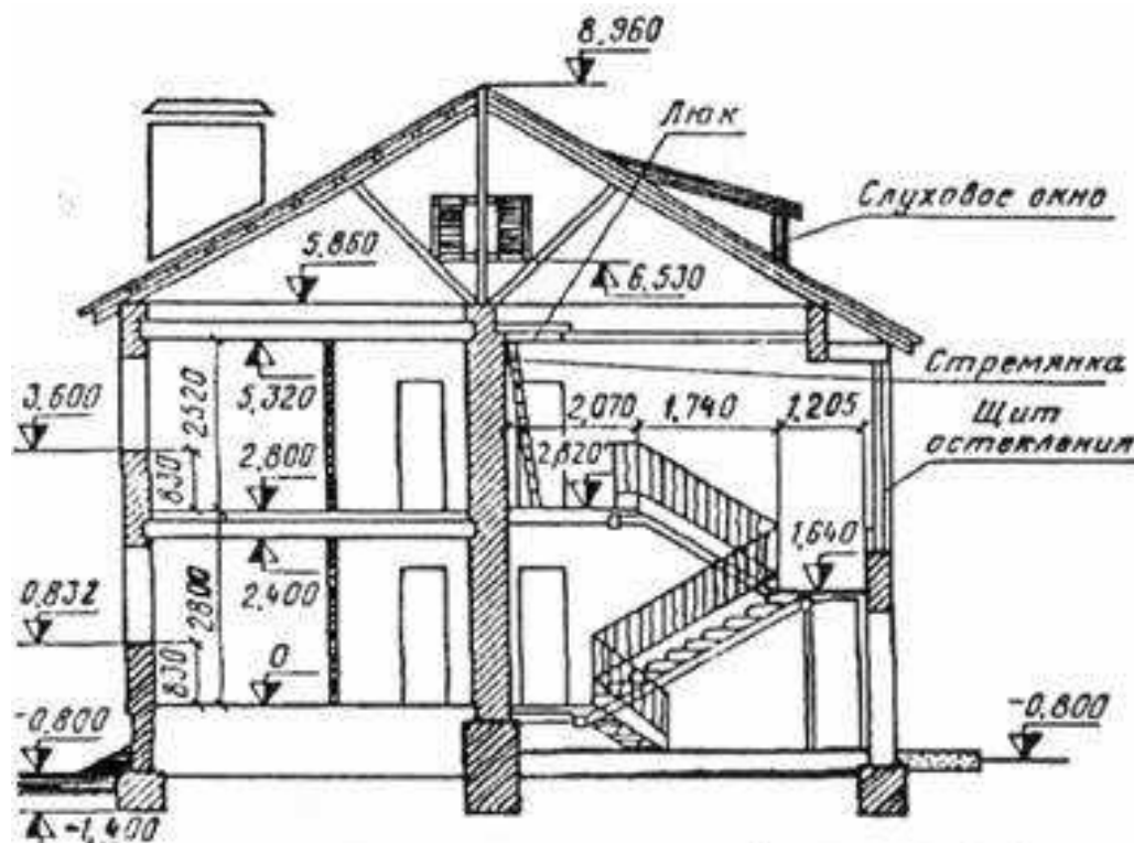
Рис. 5. Профильный план здания.
