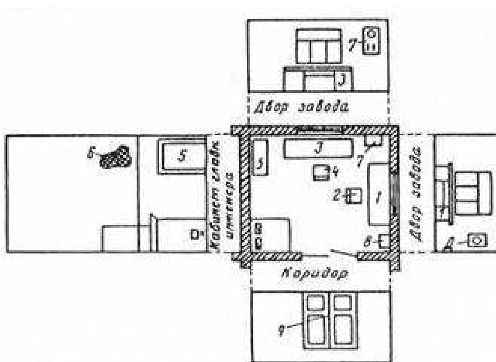
Рис. 3. Развернутый план помещения.
