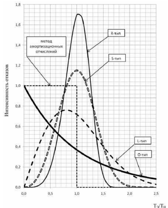
Рис. 2. Кривые интенсивности отказов O-, L-, S- и R-типа и кривая интенсивности отказов, соответствующая методу амортизационных отчислений
