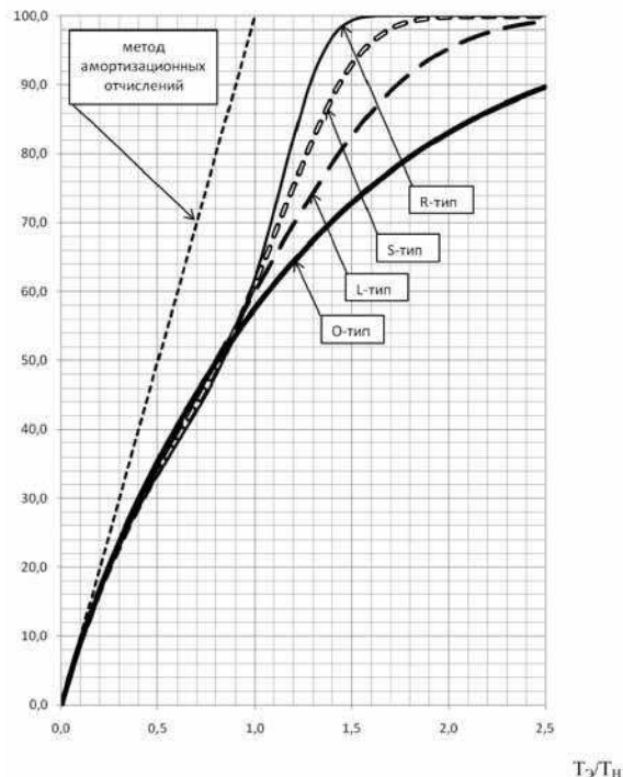
Рис. 4. Зависимости коэффициента износа от эффективного возраста, нормированного на назначенный (нормативный) срок службы, полученные различными методами
