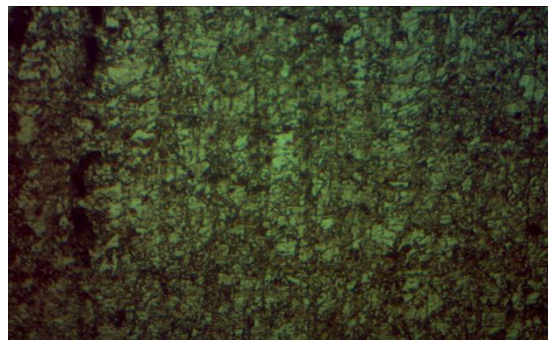
Рис. 2. Медный проводник после трех этапов травления
