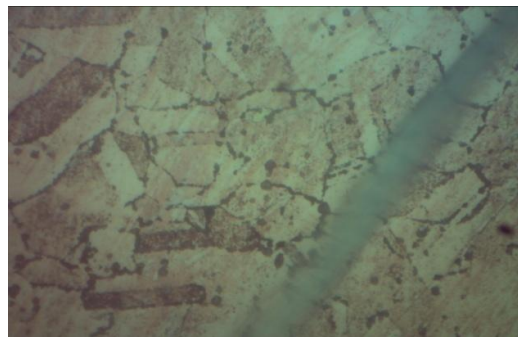
Рис. 4. Медный проводник после воздействия КЗ (увеличение 500)
