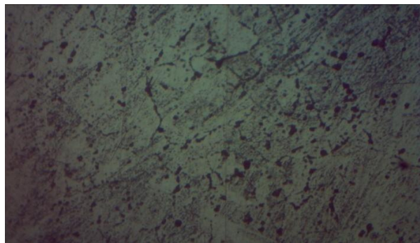
Рис. 3. Медный проводник после воздействия КЗ (увеличение 300)
