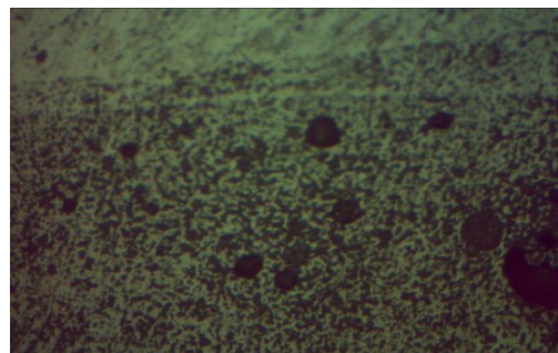
Рис. 6. Полное разрушение дендритной структуры медного проводника в зоне оплавления
