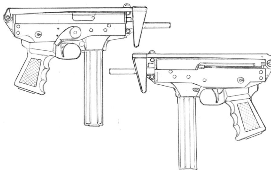
Рисунок 16 – Общий вид пистолета-пулемета ПП-91 «Кедр»
