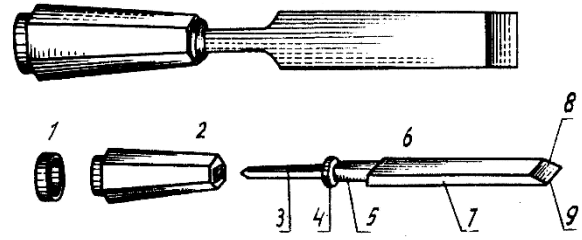
Стамеска
