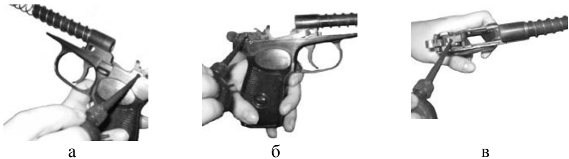
Рис. 16. Нанесение смазки: а – на цапфы шептала, б – на цапфы курка, в – на место касания курка и шептала
