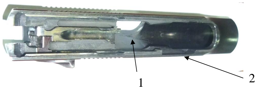
Рис. 17. Поломки на затворе ПМ: 1 – поломка досылателя, 2 – место наиболее частого образования трещины на затворе
