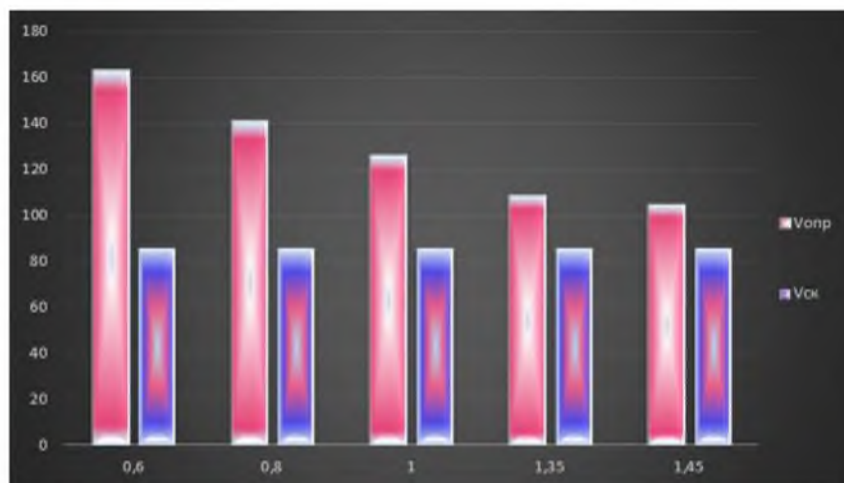
Рисунок 6. Критические скорости автомобиля «Mercedes-Benz Sprinter» на дорожном покрытии – мокрый асфальтобетон
