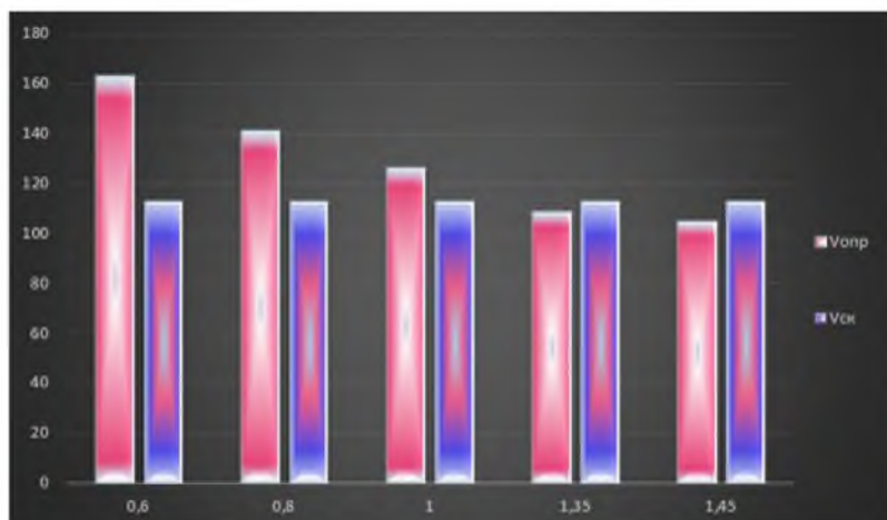
Рисунок 3. Критические скорости автомобиля «Toyota Probox I» на дорожном покрытии – сухой асфальтобетон
