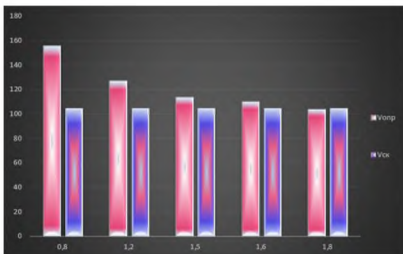
Рисунок 4. Критические скорости автомобиля «Mercedes-Benz Sprinter» на дорожном покрытии – сухой асфальтобетон
