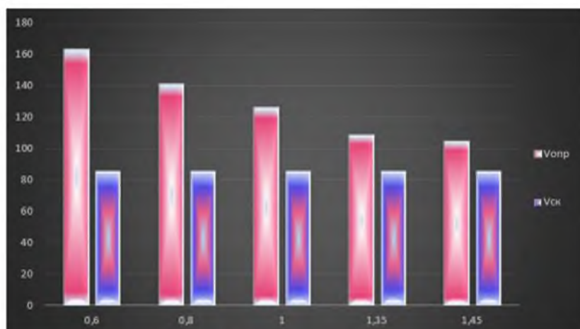
Рисунок 5. Критические скорости автомобиля «Toyota Probox I» на дорожном покрытии – мокрый асфальтобетон
