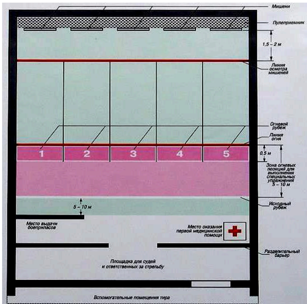
Рисунок 2. Примерная схема тира
