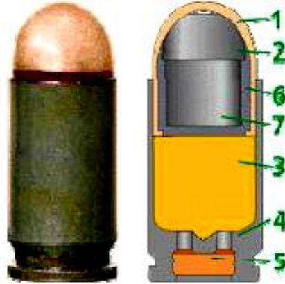
Рис. 22. Общий вид 9-мм пистолетного патрона и его устройство (1 — биметаллическая (плакированная) оболочка; 2 — пуля; 3 — пороховой заряд; 4 — гильза; 5 — капсюль; 6 — свинцовая рубашка; 7 — стальной сердечник)
