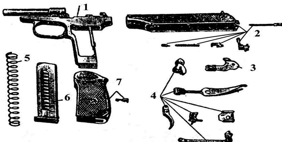
Рисунок 5. Основные части и механизмы: 1 — рамка со стволом и спусковой скобой; 2 — затвор с ударником, выбрасывателем и предохранителем; 3 — затворная задержка; 4 — ударно-спусковой механизм; 5 — возвратная пружина; 6 — магазин; 7 — рукоятка с винтом
