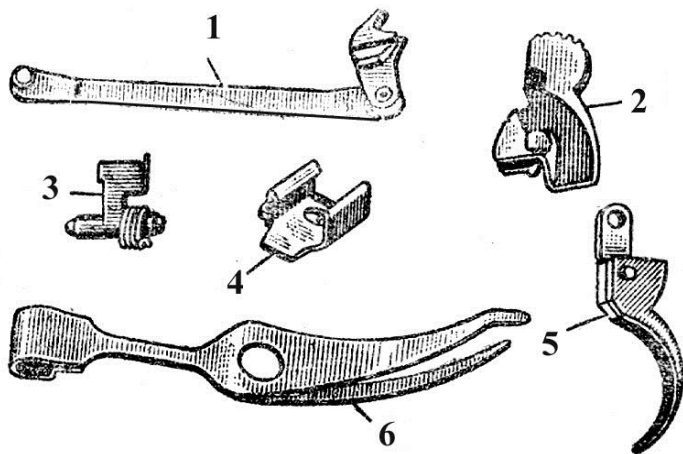
Рисунок 12. Части ударно-спускового механизма: 1 — спусковая тяга с рычагом взвода; 2 — курок; 3 — шептала с пружиной; 4 — задвижка боевой пружины; 5 — спусковой крючок; 6 — боевая пружина
