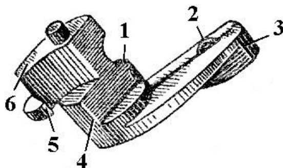
Рисунок 10. Предохранитель (1 — уступ; 2 — фиксатор; 3 — флажок предохранителя; 4 — ребро; 5 — зацеп; 6 — выступ)
