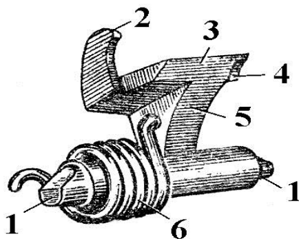
Рисунок 16. Шептало (1 — цапфы шептала; 2 — зуб; 3 — носик шептала; 4 — выступ; 5 — стойка шептала; 6 — пружина шептала)
