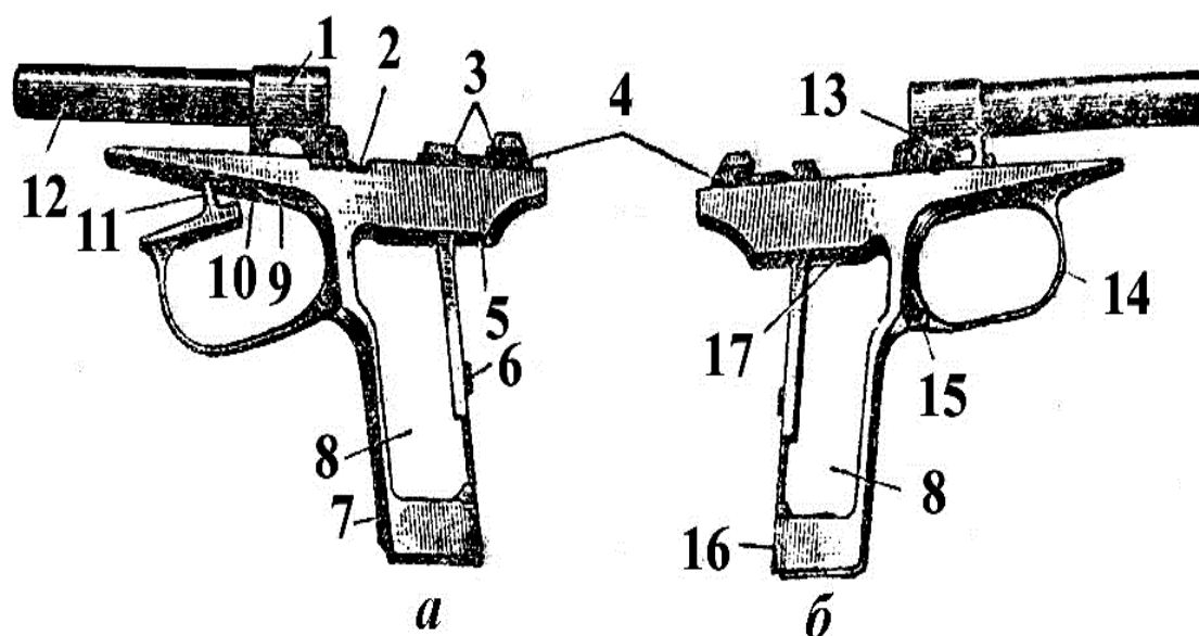
Рисунок 6. Рамка со стволом и спусковой скобой: а — левая сторона; б — правая сторона; 1 — стойка для крепления ствола; 2 — вырез для затворной задержки; 3 — цапфенные гнезда для цапф курка и шептала; 4 — пазы для направления движения затвора; 5 — окно для перьев боевой пружины; 6 — прилив с резьбовым отверстием; 7 — основание рукоятки; 8 — боковые окна; 9 — окно для размещения спускового крючка и гребня спусковой скобы; 10 — цапфенные гнезда для цапф спускового крючка; 11 — гребень для ограничения движения затвора; 12 — ствол; 13 — кривой паз для размещения и движения передней цапфы спусковой тяги; 14 — спусковая скоба; 15 — прилив с гнездом для крепления спусковой скобы; 16 — вырез для защелки магазина; 17 — окно для выхода верхней части магазина [6]
