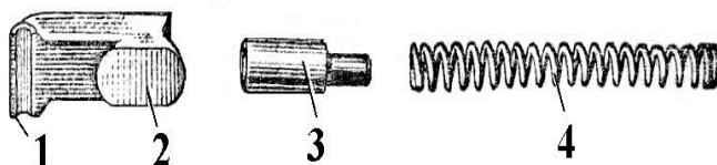
Рисунок 9. Выбрасыватель (1 — зацеп; 2 — пяточка для соединения с затвором; 3 — гнеток; 4 — пружина выбрасывателя)
