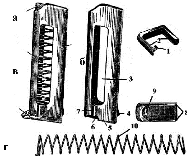
Рисунок 20. Магазин (а — подаватель; б — корпус магазина; в — пружина подавателя; г — крышка магазина; 1 — зуб; 2 — отогнутые концы; 3 — окно; 4 — выступ; 5 — загнутое ребро; 6 — вырез; 7 — желоб; 8 — пазы; 9 — отверстие; 10 — пружина подавателя)
