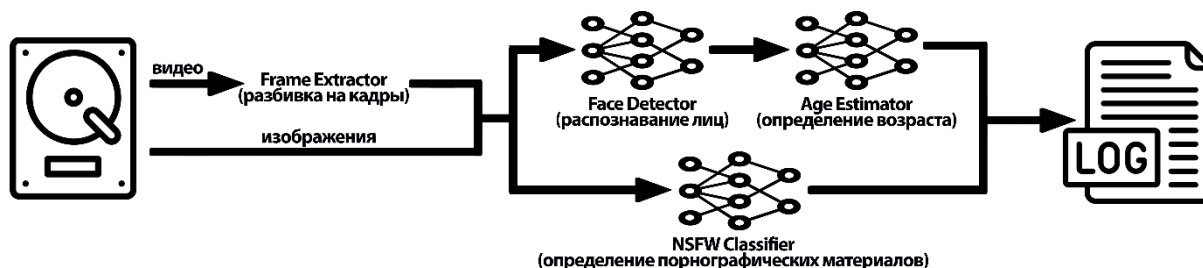
Рис. 1. Схема конвейерной обработки цифровых данных для выявления файлов с детской порнографией
