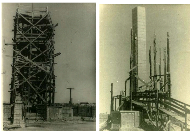
Рис. 7. Строительство пилона
