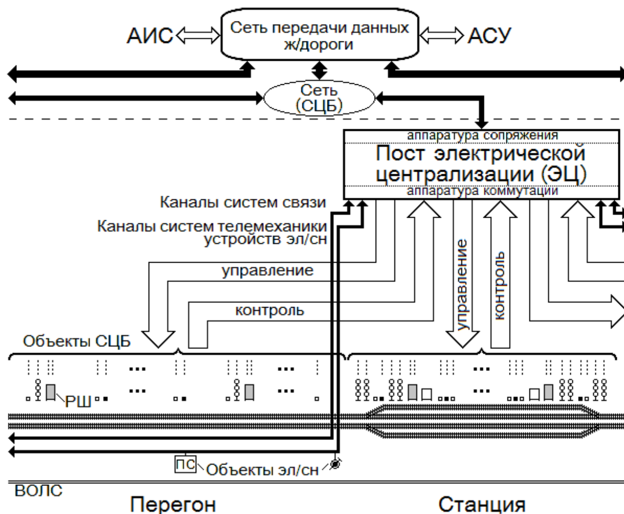
Рис. 1. Структурная схема передачи информации между объектами перегонов и станций и сетью передачи данных железной дороги
