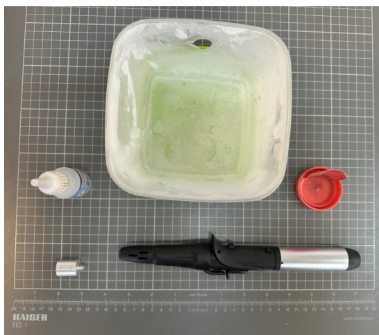
Рис. 1. Цианакрилатный генератор, емкость с клеем, гильза и герметичная камера (контейнер) для выявления следов рук
