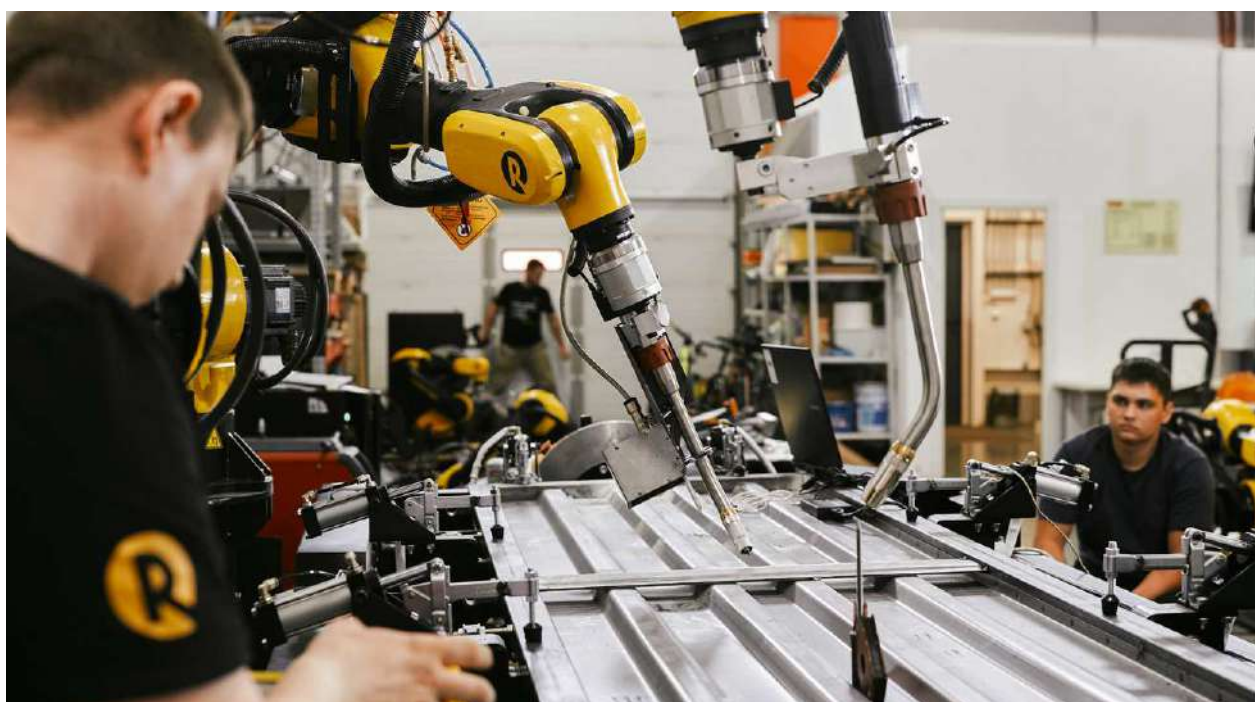
Роботизированная сварочная ячейка A12-PVHH-600.
