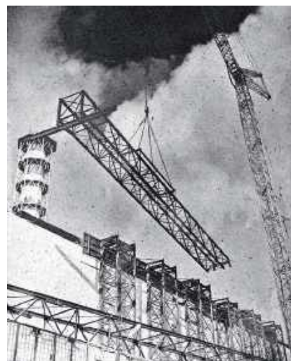
МОНТАЖ ОПОР ДЛЯ СООРУЖЕНИЯ УКРЫТИЯ НАД 4-М ЭНЕРГОБЛОКОМ, 1986 ГОД
