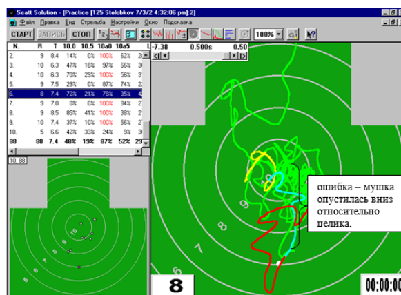
Рис. 2. Пример цветовой дифференциации ошибки прицеливания на тренажере СКАТТ
