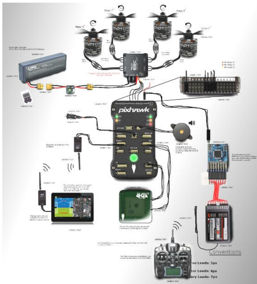
Рис. 1. Компоненты беспилотного летательного аппарата
