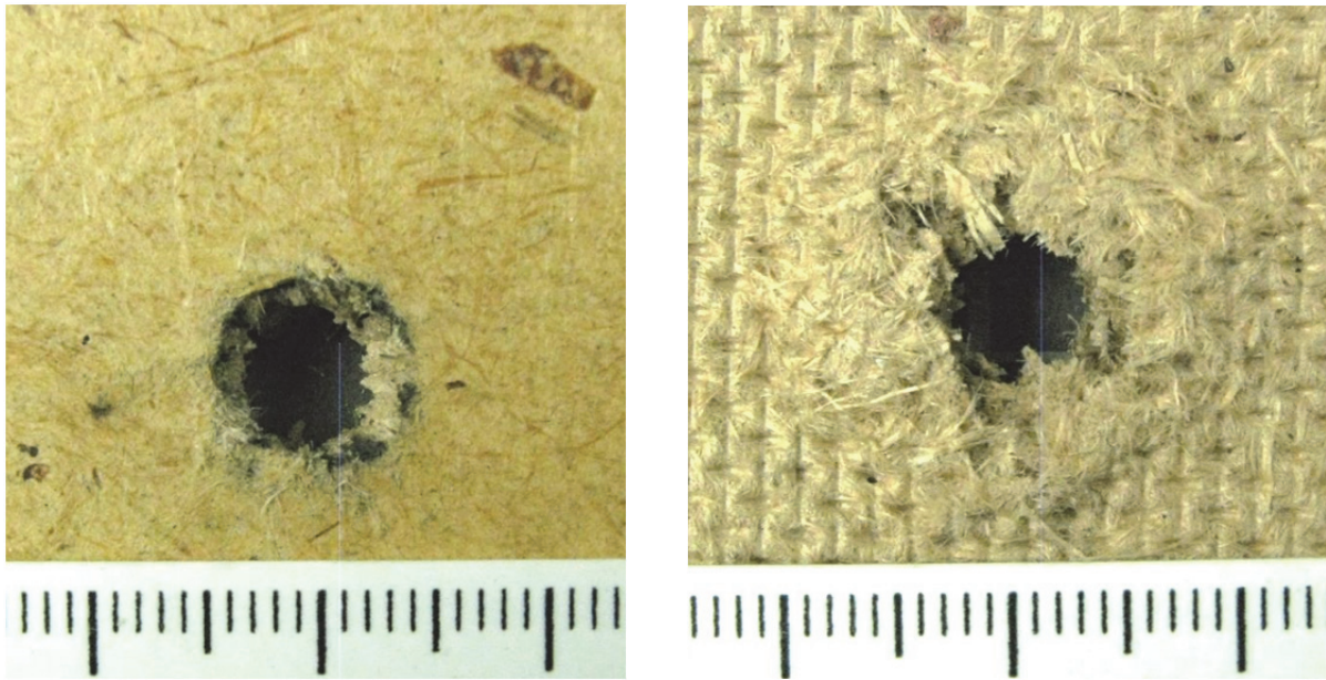
Рис. 5. Входное (слева) и выходное (справа) отверстия на древесно-волоконистой плите толщиной 3 мм (угол 90^\circ , дистанция 30 см)
